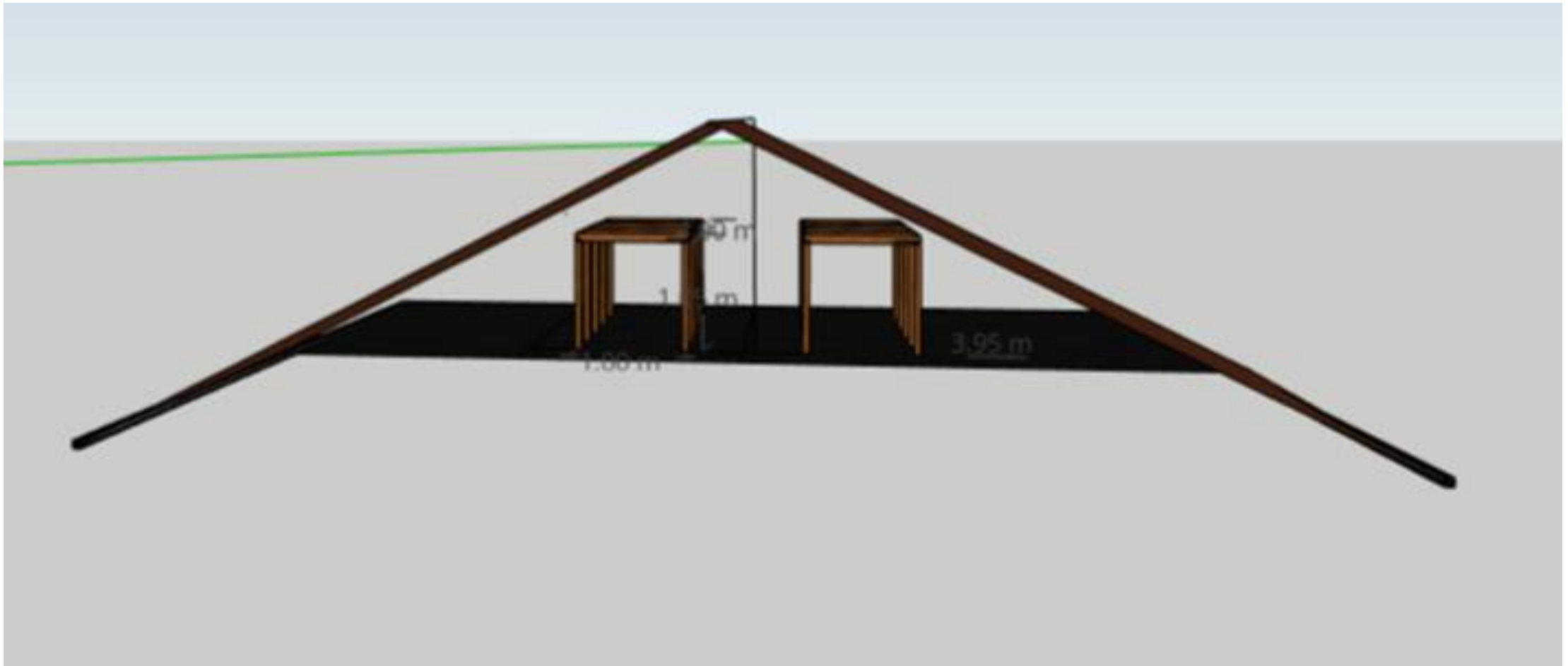
Figura 12. Vista frontal secadora con techo corredizo. Fuente : del autor.
