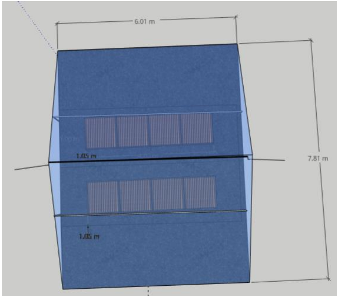
Figura 9. Vista superior secadora tipo a dos aguas. Fuente : del autor.
