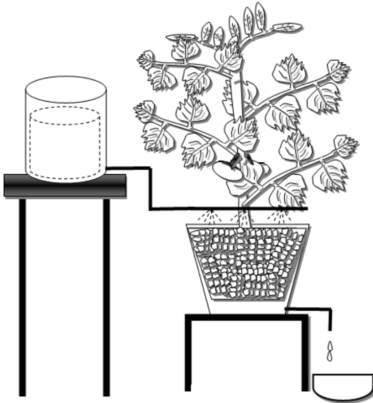
Figura 1: Componentes generales de la hidroponía
