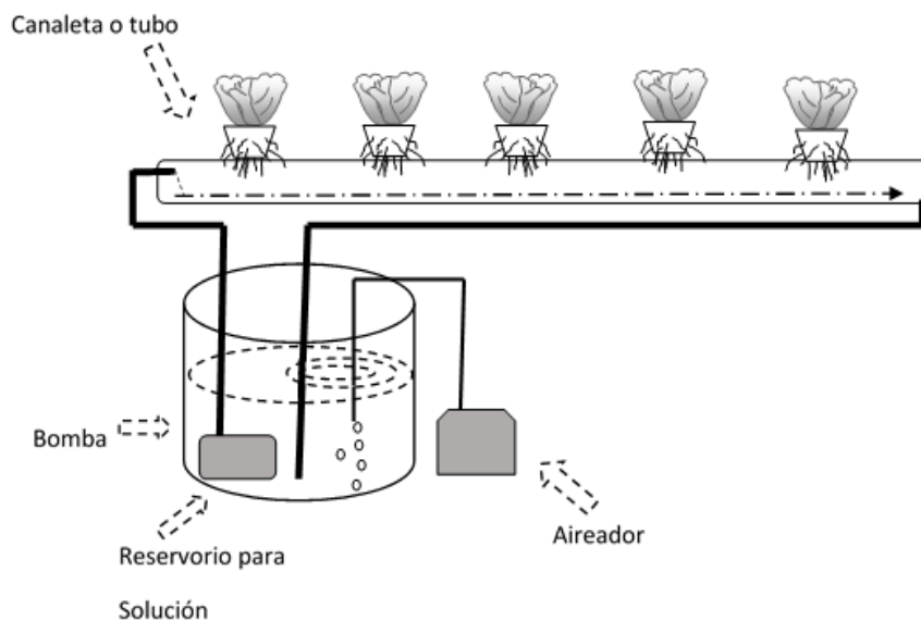
Figura 33: Modelo básico de un sistema NFT
