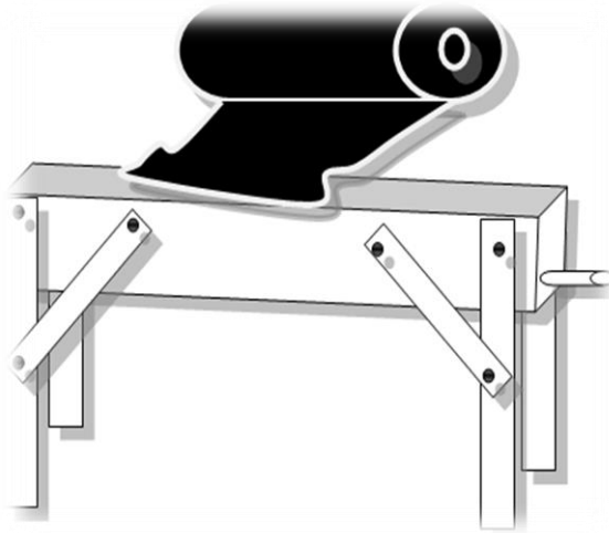
Figura 23: Cama de madera con plástico para impermeabilizar
