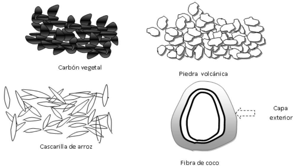
Figura 15: Algunos materiales empleados como sustratos
